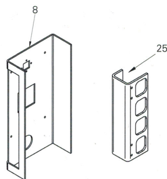
DETTAGLIO PIASTRA SERRATURA
