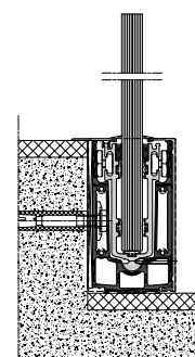
Soluzione con fissaggio a pavimento/muro
